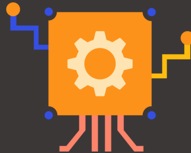
Malware
